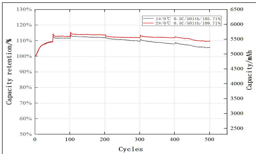
6.0 Ah 磷酸铁锂电池 0±2℃ 0.5C 循环曲线图 (A+/A) 0±2℃ 0.5C cycle curve of 6.0 Ah LiFePO 4 cell (A+/A)
