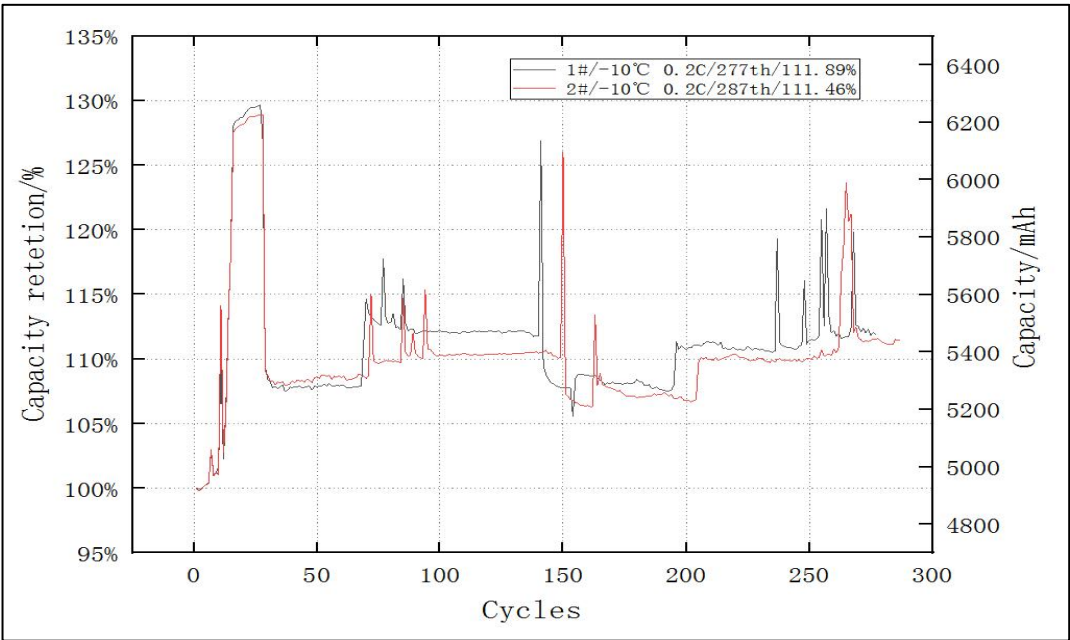
6.0 Ah 磷酸铁锂电池 -10±2℃ 0.2C 循环曲线图 (A+/A) -10±2℃ 0.2C cycle curve of 6.0 Ah LiFePO 4 cell (A+/A)
