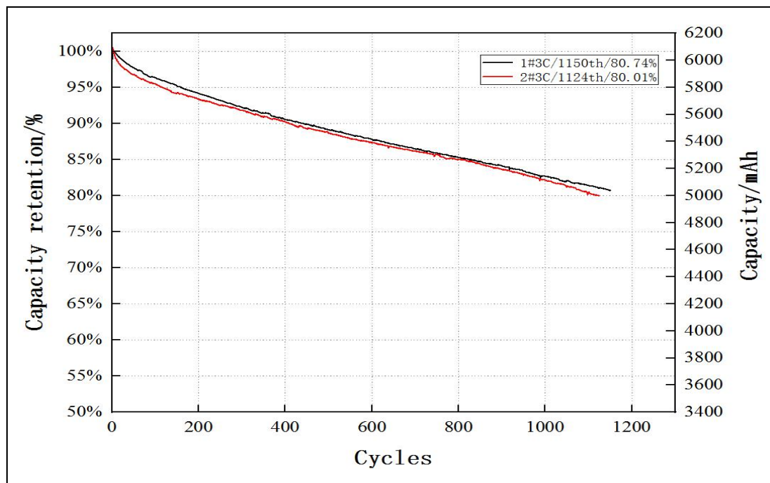
6.0 Ah 磷酸铁锂电池 30±2℃ 3C 循环曲线图 30±2℃ 3C cycle curve of 6.0 Ah LiFePO 4 cell
