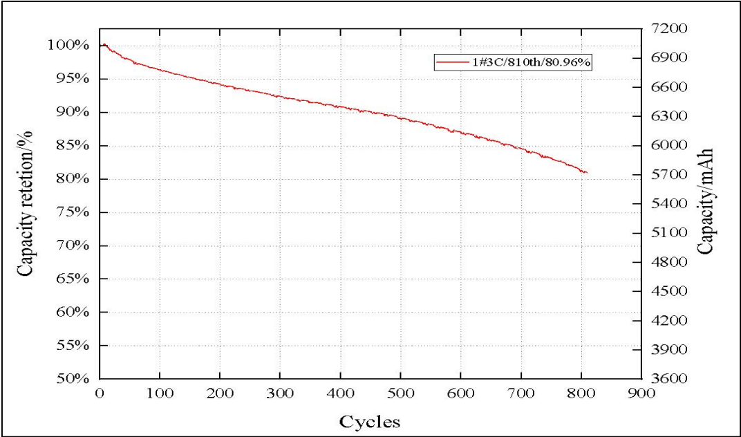
7.0 Ah 磷酸铁锂电池 30±2℃ 3C 循环曲线图 30±2℃ 3C cycle curve of 7.0Ah LiFePO 4 cell
