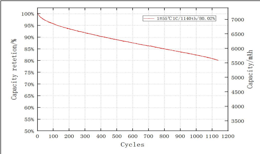
7.0 Ah 磷酸铁锂电池 55±2℃ 1C 循环曲线图 55±2℃ 1C cycle curve of 7.0 Ah LiFePO 4 cell
