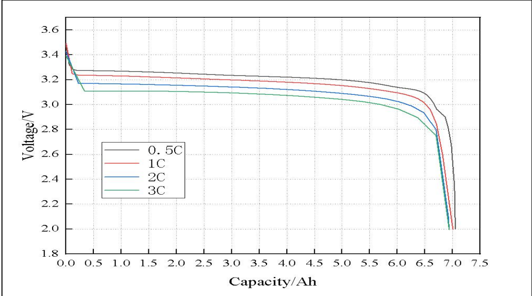
7.0Ah 磷酸铁锂系电池不同倍率放电曲线 Different rate discharge curve of 7.0Ah LiFePO 4 cell
