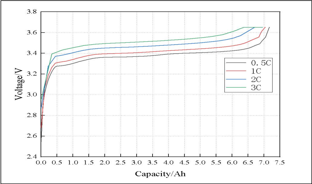
7.0Ah 磷酸铁锂系电池不同倍率充电曲线 Different rate charge curve of 7.0Ah LiFePO 4 cell
