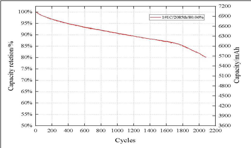
7.0 Ah 磷酸铁锂电池 30±2℃ 1C 循环曲线图 30±2℃ 1C cycle curve of 7.0Ah LiFePO 4 cell
