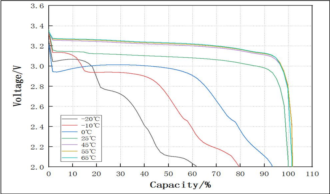
7.0 Ah 磷酸铁锂电池不同温度放电曲线（1C） Discharge curve of 7.0 Ah LiFePO 4 cell at different temperatures(1C)
