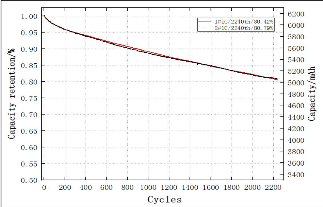
6.0 Ah 磷酸铁锂电池 30±2℃ 1C 循环曲线图（A+） 30±2℃ 1C cycle curve of 6.0Ah LiFePO 4 cell（A+）
